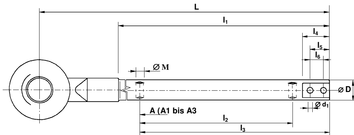
Zugöse DIN 74054-40 C
